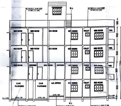
SECTION-BB SCALE: 1:100
