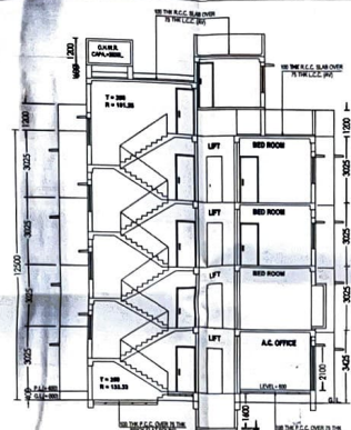
SECTION-AA SCALE: 1:100
