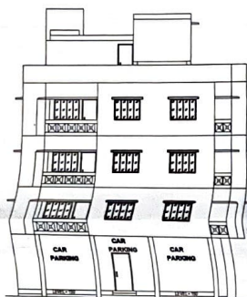
FRONT SIDE ELEVATION SCALE: 1:100
